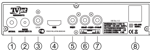
Рис.2 Задняя панель приемника
