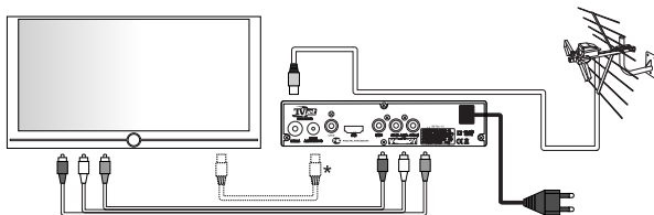
Рис.7 Схема подключения уличной антенны
