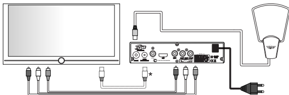
Рис.6 Схема подключения комнатной антенны
