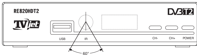
Рис.4 Зона приема команд ПДУ
