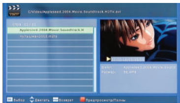
Рис 33. Выбор видеофайла.
