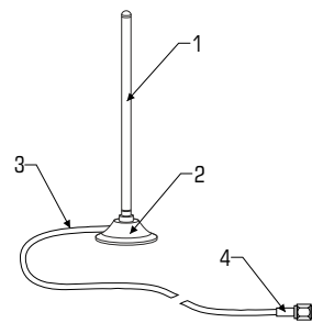
Рис.2 Устройство антенны
